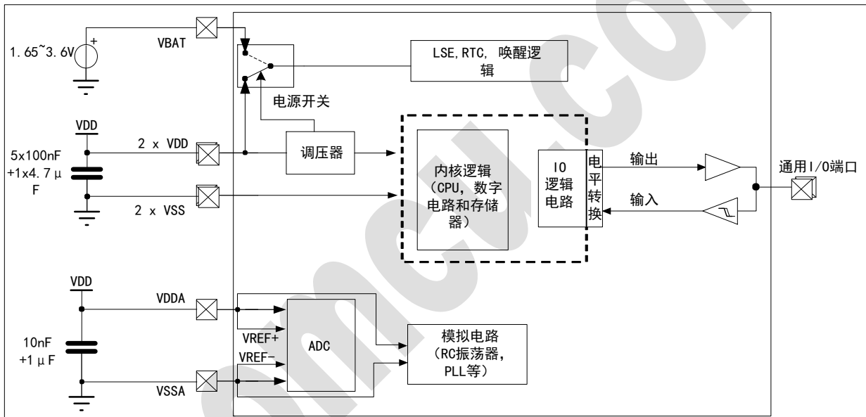
供电方案
