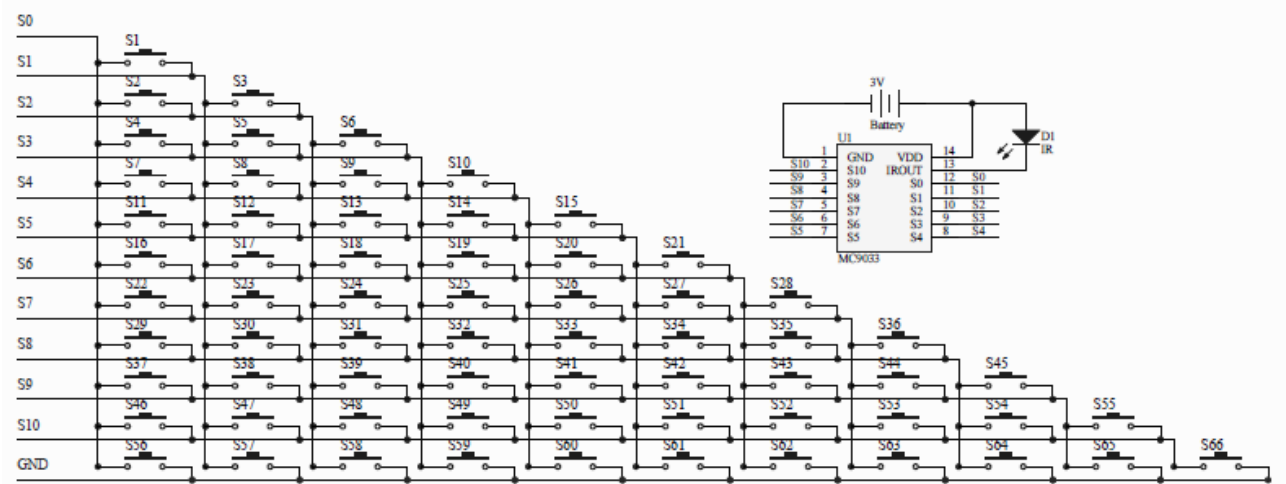
66 键 原理图
